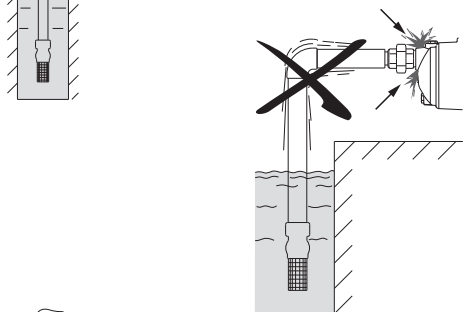
Fig. 4 Sostegni ed ancoraggi delle tubazioni Supports and clamps for pipelines Stützen und Verankerungen der Rohrleitungen Soutien et ancrage des tuyaux Sostén y anclaje de la instalación Konsoll samt klämmor för rör Steunen voor leidingen Υποστήριξη και σφίξιμο σωληνώσεων Опоры и крепления труб 管路的支撑与紧固
