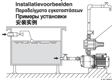
Fig. 2 Funzionamento sotto battente Positive suction head operation Zulaufbetrieb Fonctionnement en charge Funcionamiento bajo carga Tilrrinning sugsidan Toeloopsituatie Θέση λειτουργίας με θετική αναρρόφηση Работа под гидравлическим напором 入口正压头
